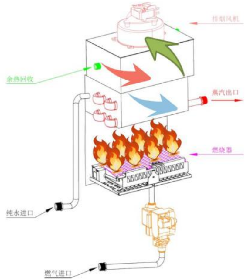
主机采用惯流交换换热原理
