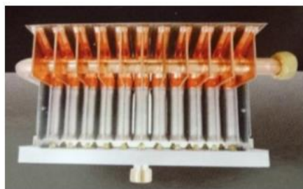
多孔燃烧器
